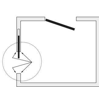
ALUMINIOWE PROFILE STARTOWE W KASETACH ECLISSE SYNTESIS LINE ORAZ SYNTESIS LUCE
