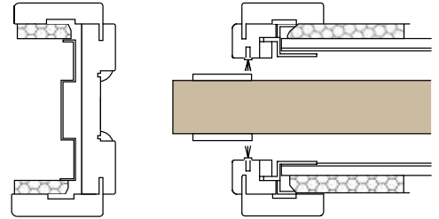
Wersja bez tunelu
