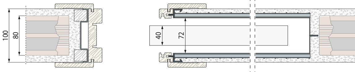
Do mokrego tynku, całkowita grubość ściany 100 mm, Ce = 80 mm
