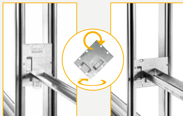
Dystans: TH 100 mm
