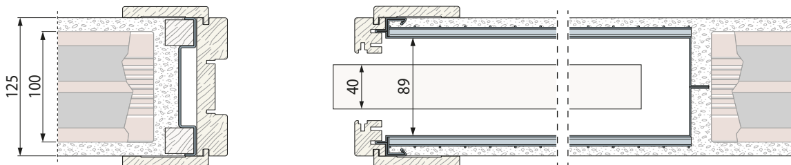
Do mokrego tynku, całkowita grubość ściany 125 mm, Ce = 100 mm
