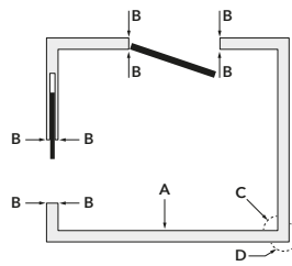
ŁĄCZNIK NAROŻNY WEWNĘTRZNY
