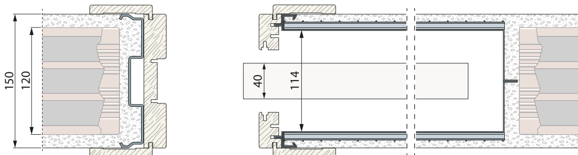
Do mokrego tynku, całkowita grubość ściany 150 mm, Ce = 120 mm
